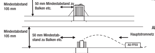
Abb.1 Vorderansicht
